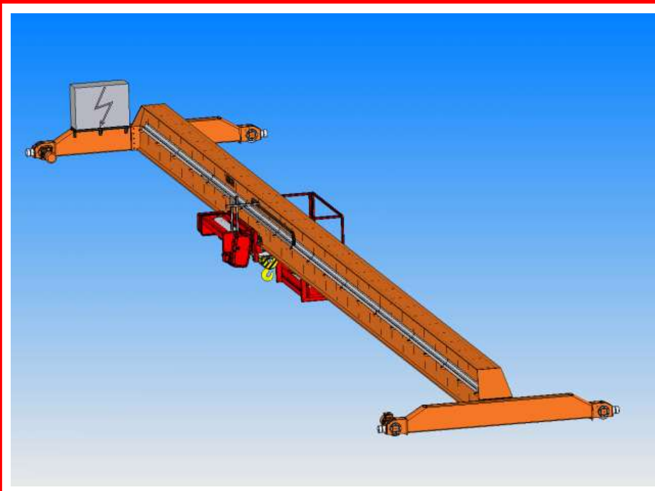
■ Однобалочный мостовой кран тип GJMJ 5t/21,5m с платформой для обслуживания на тельфере
