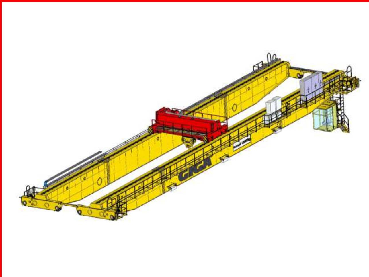
■ Двухбалочный мостовой кран тип GDMJ 120t/50t/41,25m
