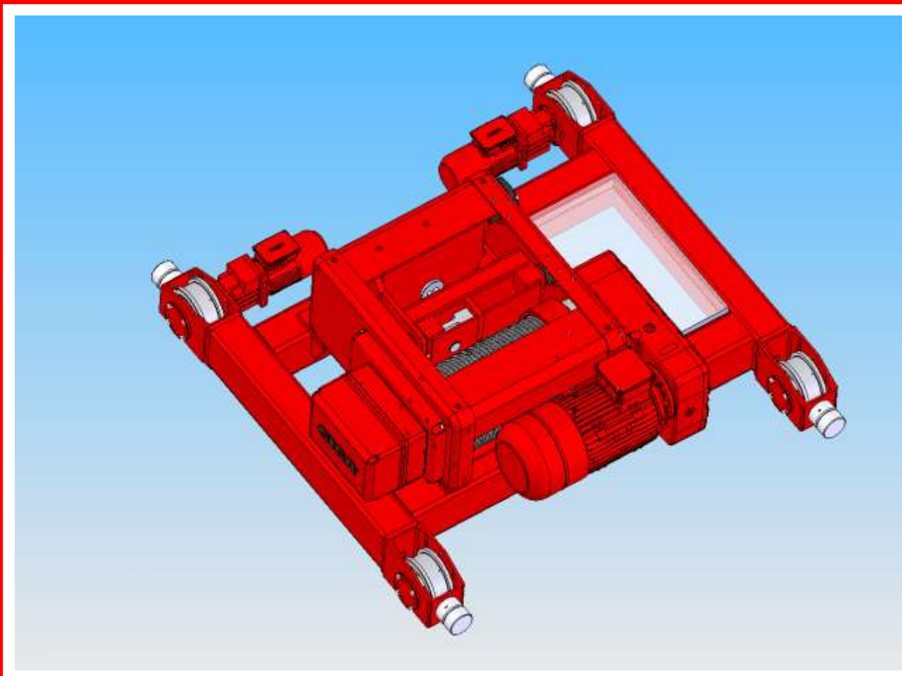
■ Электрический канатный тельфер 20т тип GHM20000-16-4/1-6M,D
