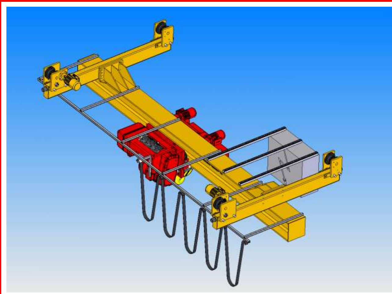
Подвесной мостовой кран тип GPMJ 5t/6m
