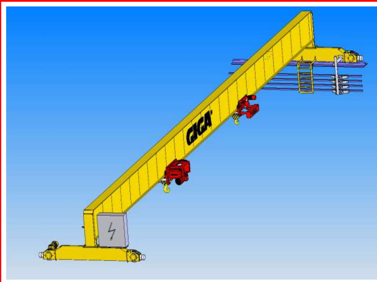
■ Однобалочный мостовой кран тип GJMJ 12,5t/5t/24m
