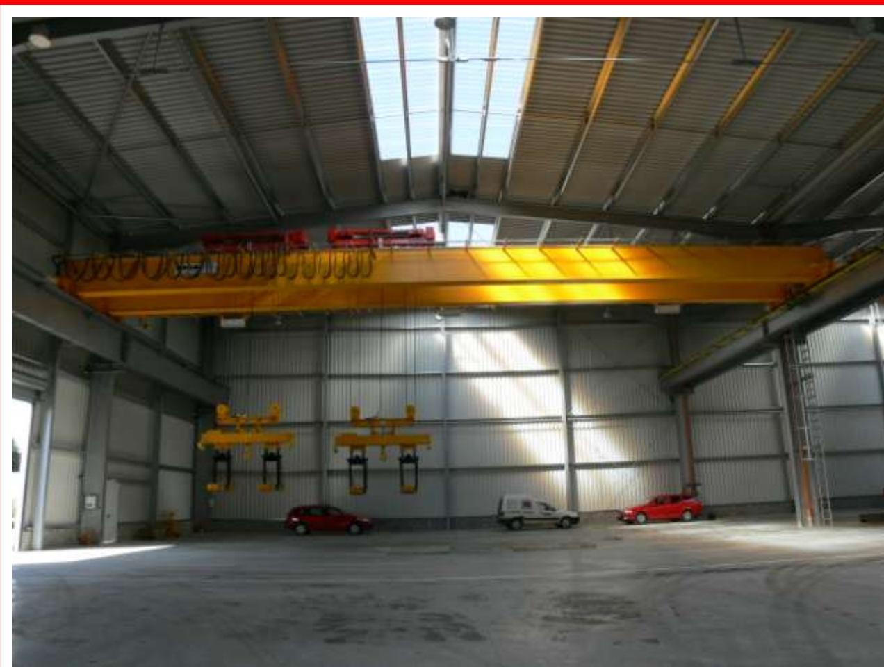
■ Двухбалочный мостовой кран тип GDMJ 2x10t/25,5m с канатной стабилизацией на магнитном траверсе
