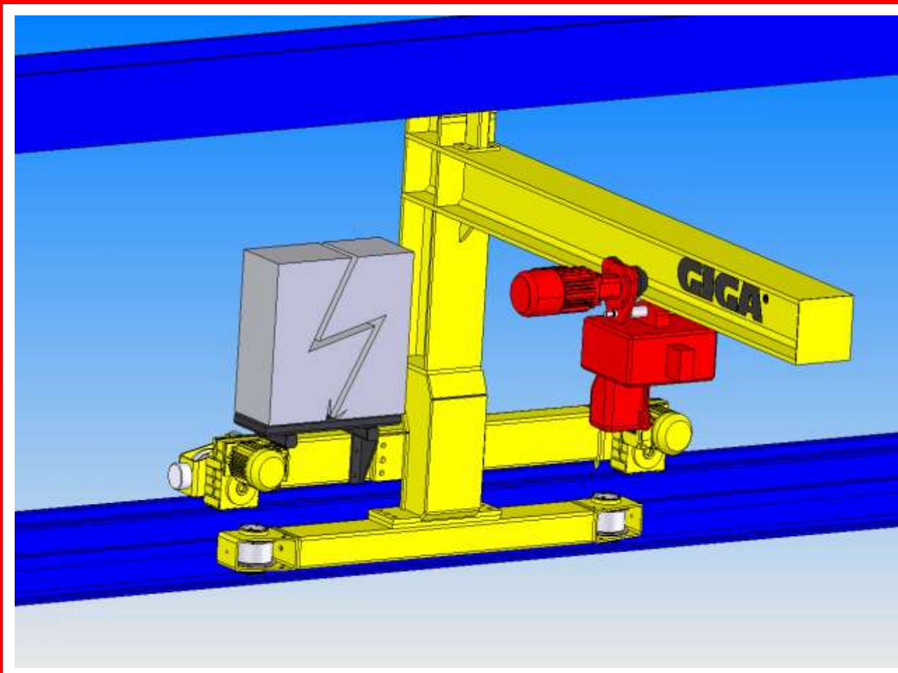
■ Консольный мостовой кран тип GKMJ 0,16t/2,5m
