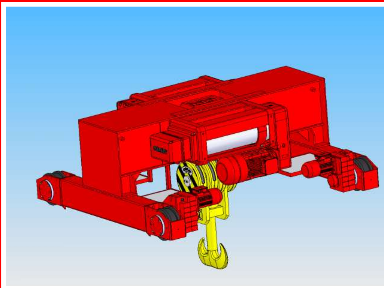
■ Электрический канатный тельфер 50т тип GHM50000-14-2x4/1-9M,D
