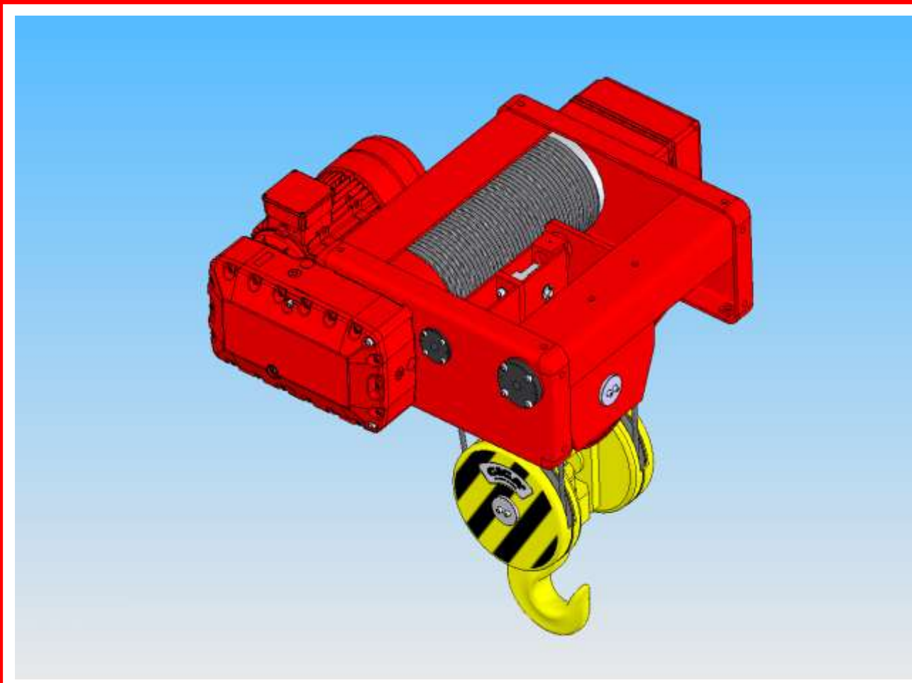
■ Электрический канатный тельфер 25т тип GHM25000-14-4/1-6M,S
