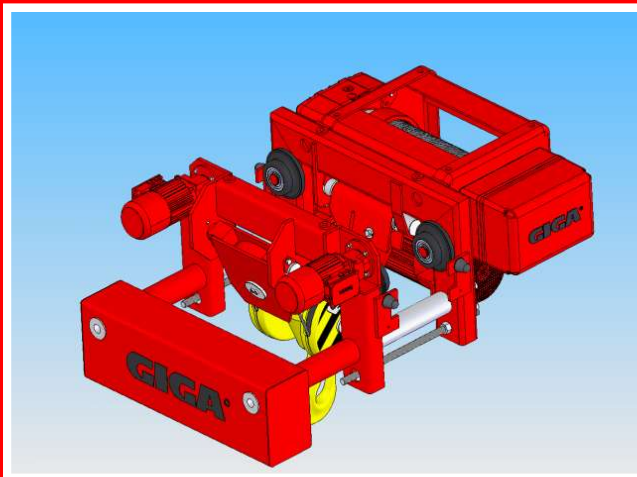
■ Электрический канатный тельфер 10т тип GHM10000-20-4/1-6M,Z
