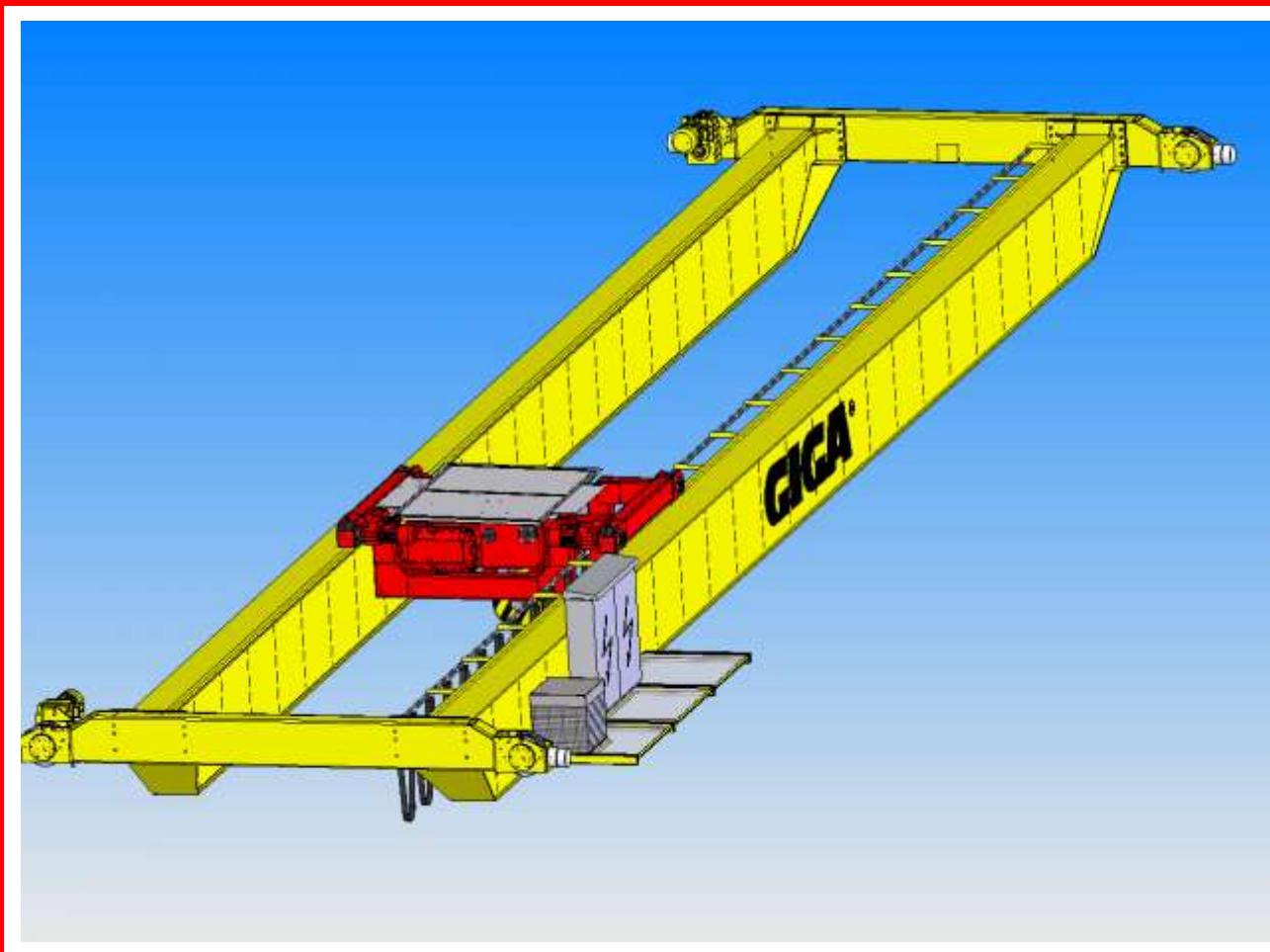
■ Двухбалочный мостовой кран тип GDMJ 15t/19,2m
