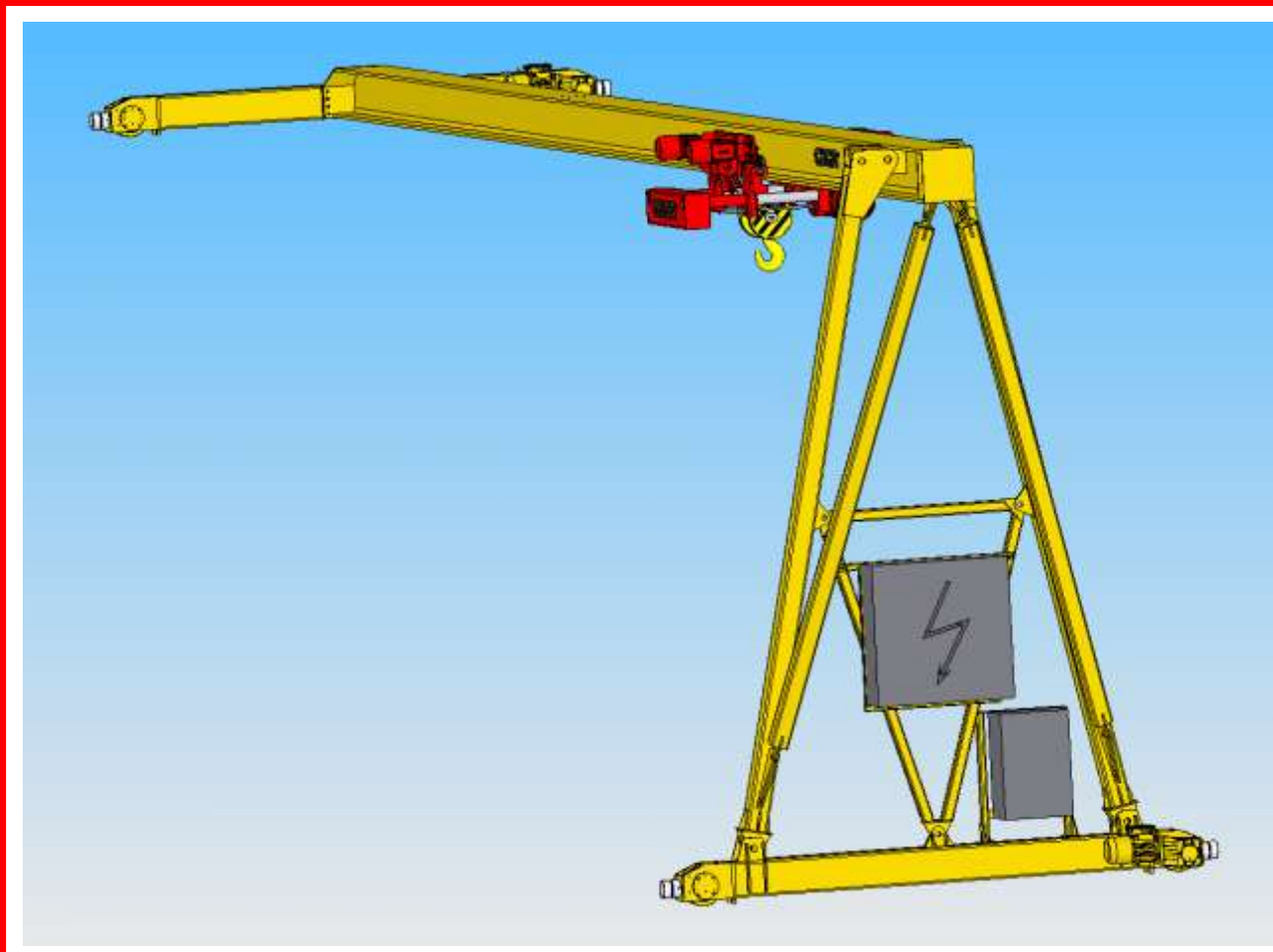
■ Полукозловой мостовой кран тип GPMJ 5t/9,5m
