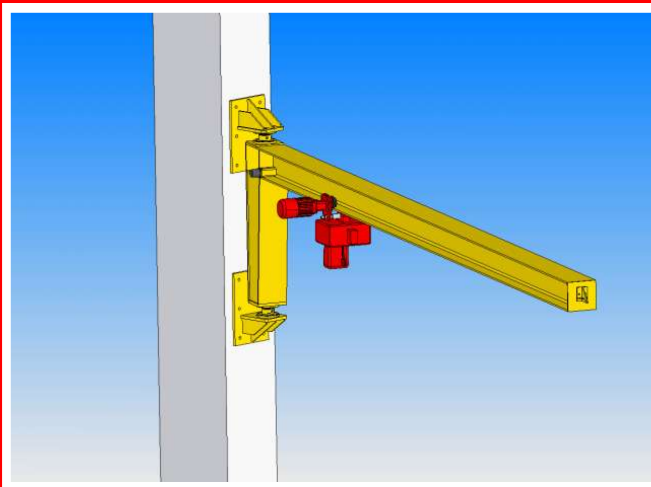
■ Консольный поворотный кран тип GKOJ 1t/4,5m
